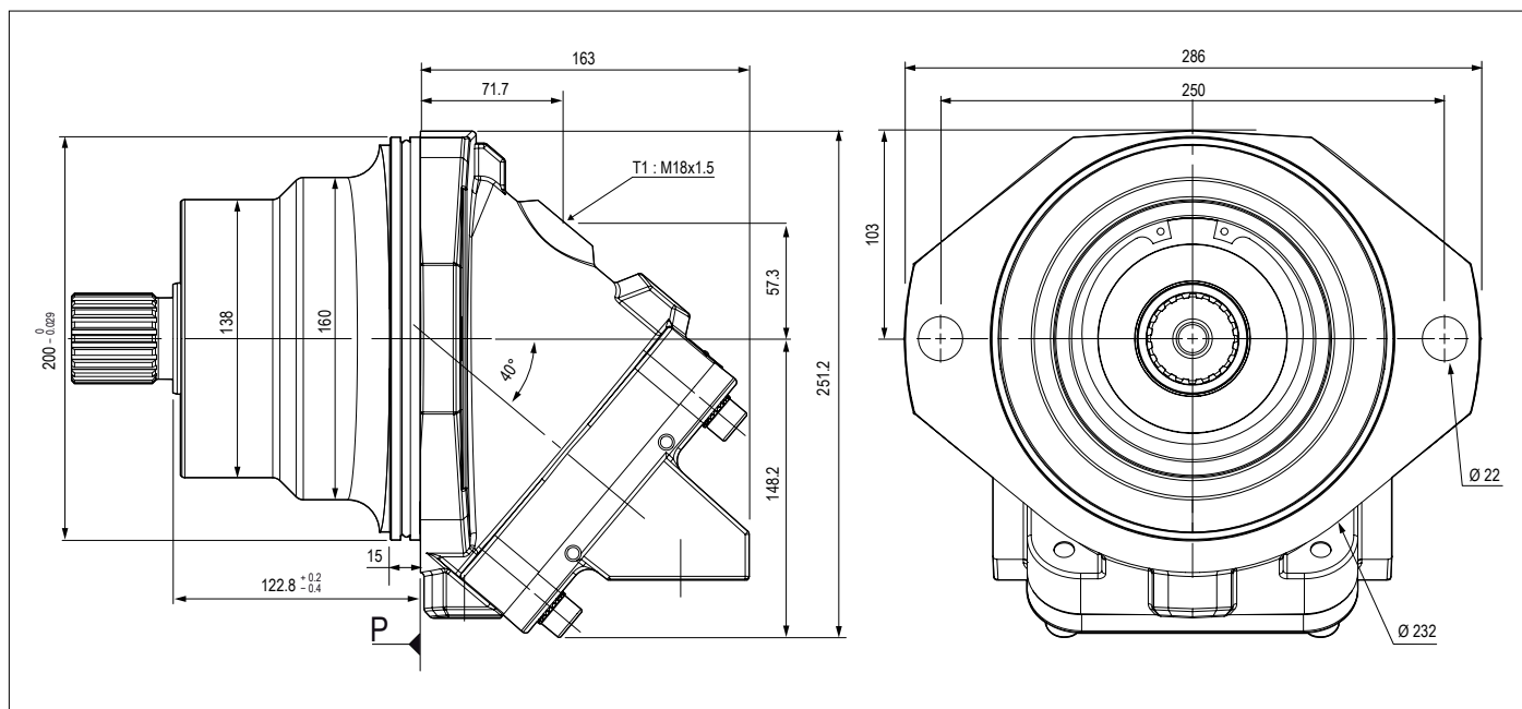
W1 花键轴 DIN 5480 W 45 x 2 x 30 x 21 x 9 g
