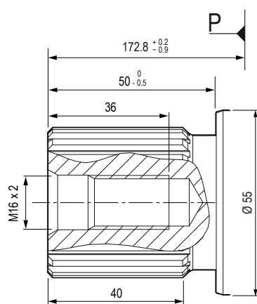
W1 花键轴 DIN 5480 W 45 x 2 x 30 x 21 x 9 g
