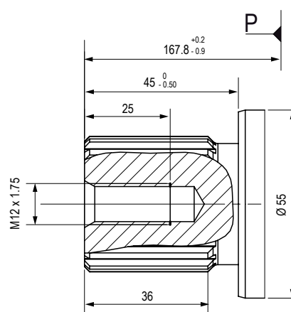
W2 花键轴 DIN 5480 W 40 X 2 X 30 X 18 X 9 g
