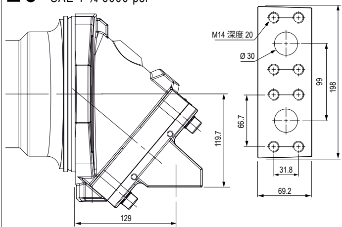
L0 SAE 法兰油口, 底部 40°, A和B SAE 1"¼ 6000 psi
